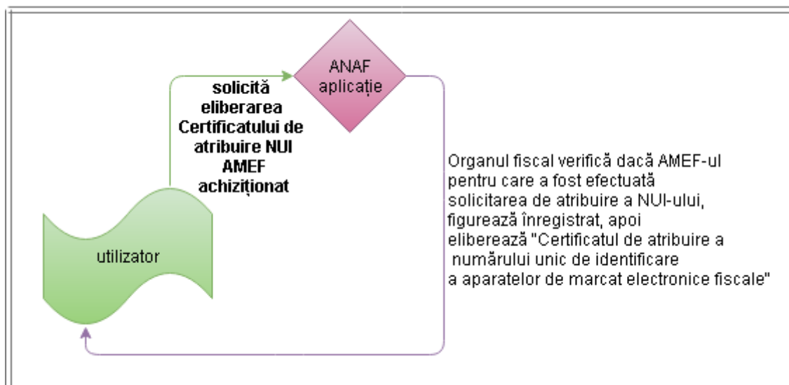
Fig.3 Diagrama procesului de solicitare și emiteră a certificatului de atribuire a numărului unic de identificare a aparatelor de marcat electronice fiscale
